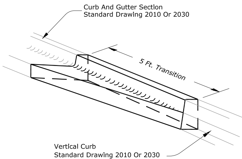
CURB TYPE TRANSITION DETAIL N.T.S.
