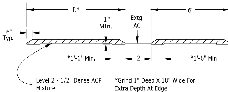
SECTION VIEW B - B N.T.S.
